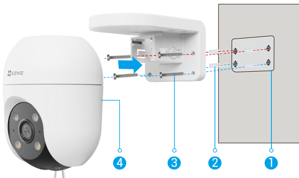
Рисунок 2. Монтаж на стену
