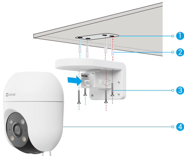
Рисунок 1. Монтаж на потолок
